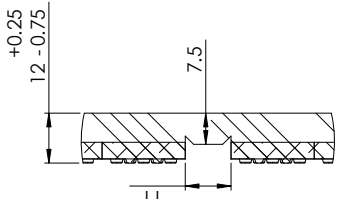
DETAIL B, TYP. SCALE 1:1
